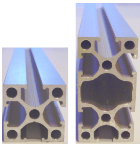
25er Profreihe
