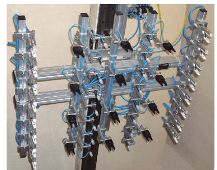
Handlingsysteme
